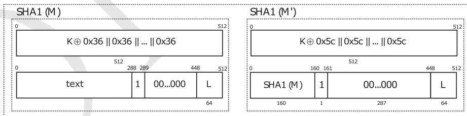
Fig. 1. HMAC-SHA-1
