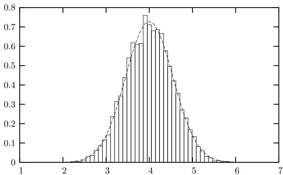
Figura 6: Verifica empirica del teorema centrale della statistica.
