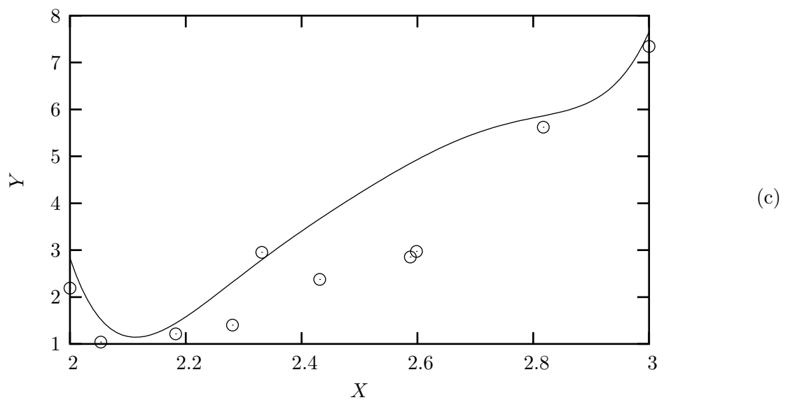
Figura 12: Confronto tra un nuovo campione di dati e le approssimazioni ottenute precedentemente: una retta (a), una parabola (b) e un polinomio di grado 6 (c)
