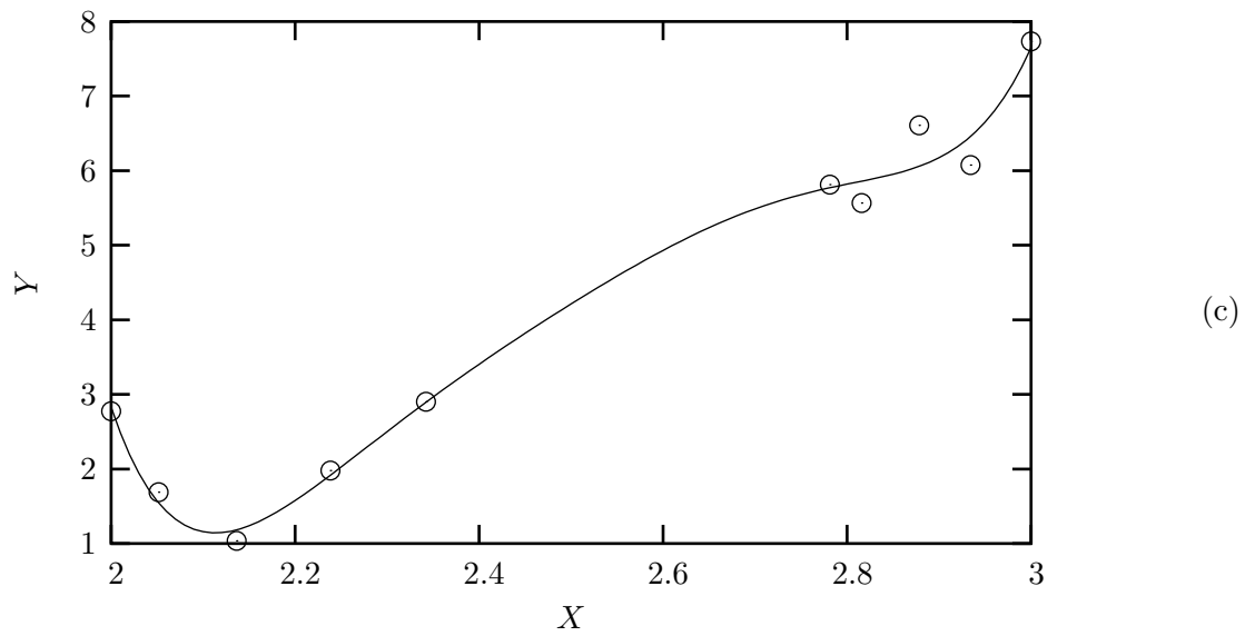
Figura 11: Approssimazione dei dati campionati con una retta (a), con una parabola (b) e con un polinomio di grado 6 (c)
