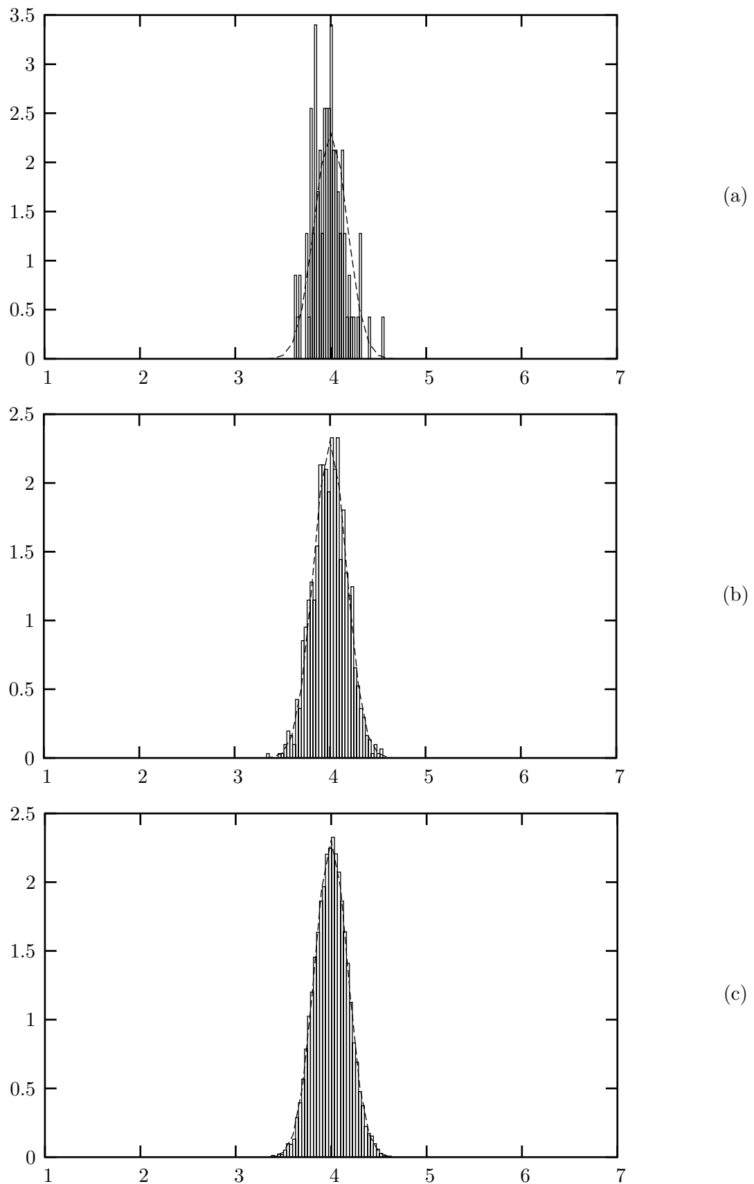
Figura 7: Verifica empirica del teorema centrale della statistica: al crescere del numero di campioni, la distribuzione della media campionaria si addensa sempre più intorno alla media della distribuzione campionata.
