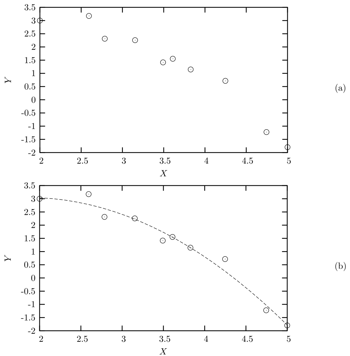
Figura 10: Esempio di un problema di regressione non lineare.
