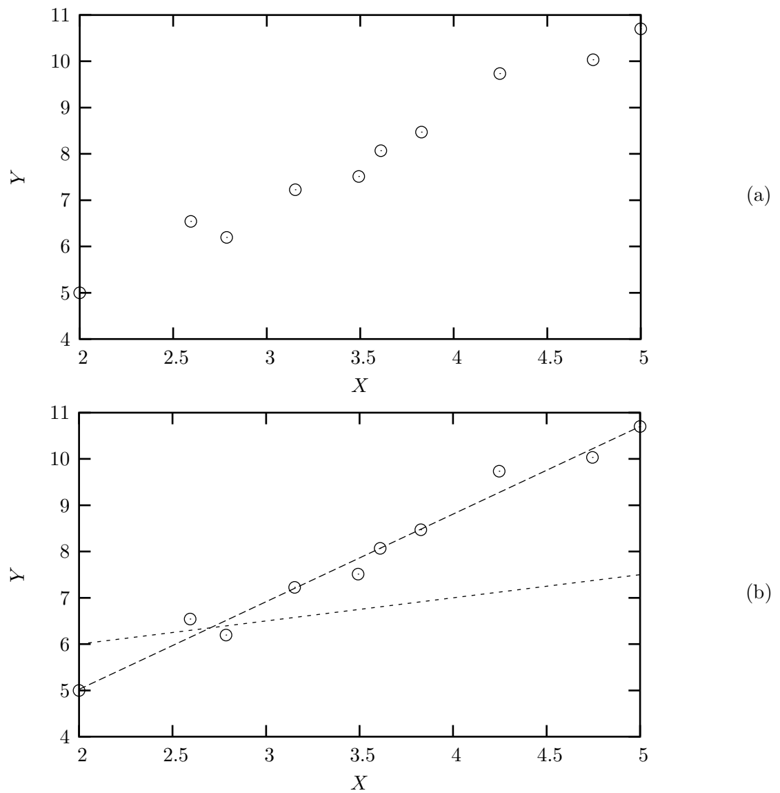
Figura 8: Esempio di un problema di regressione lineare.
