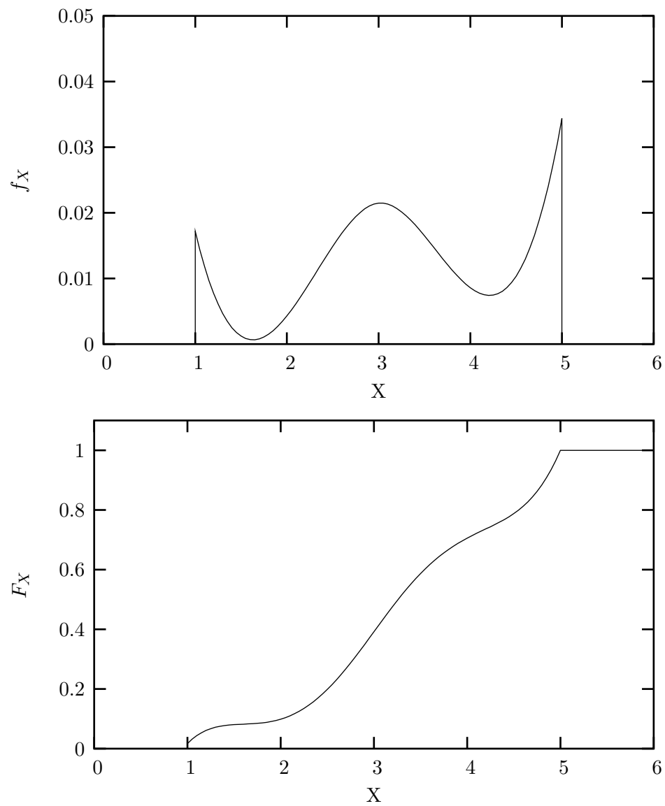
Figura 2: Distribuzione continua
