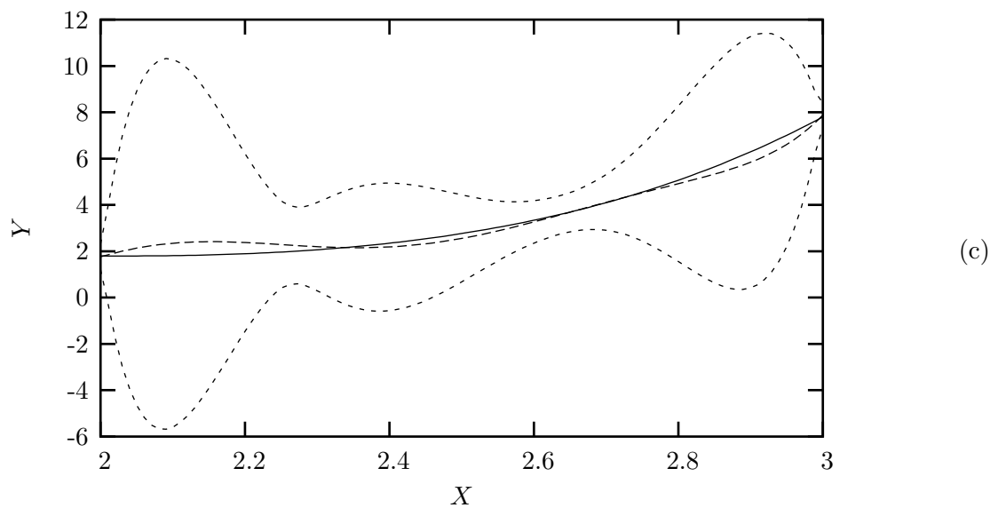
Figura 13: Bias-variance dei regressori: retta (a), parabola (b) e polinomio di grado 6 (c). La linea continua, quella a tratto lungo e quelle a tratto corto rappresentano, rispettivamente, la vera curva di regressione, l'approssimatore medio e l'ampiezza della deviazione standard degli approssimatori.
