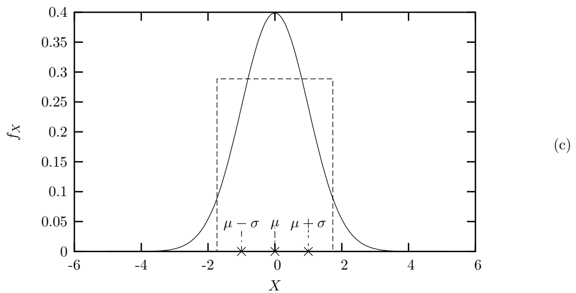
Figura 3: Media e varianza
