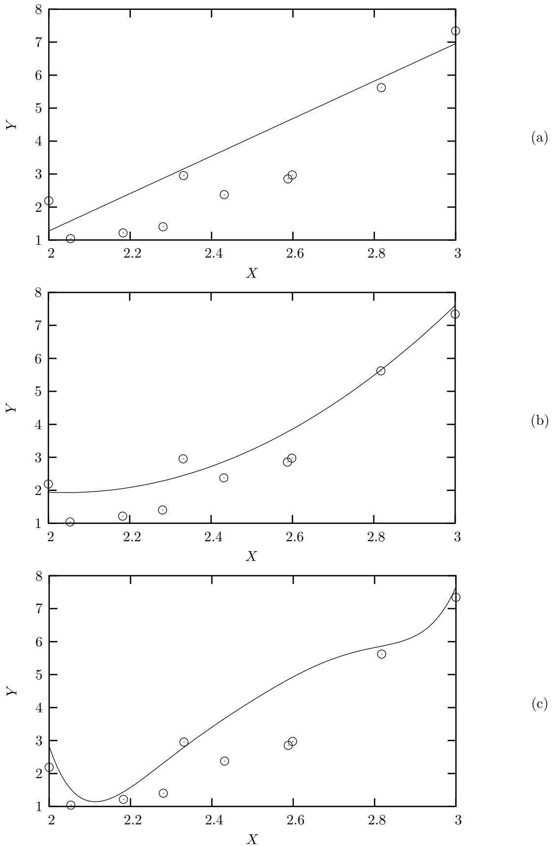
Figura 12: Confronto tra un nuovo campione di dati e le approssimazioni ottenute precedentemente: una retta (a), una parabola (b) e un polinomio di grado 6 (c)
