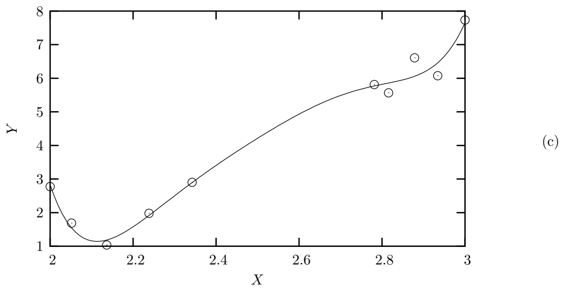
Figura 11: Approssimazione dei dati campionati con una retta (a), con una parabola (b) e con un polinomio di grado 6 (c)
