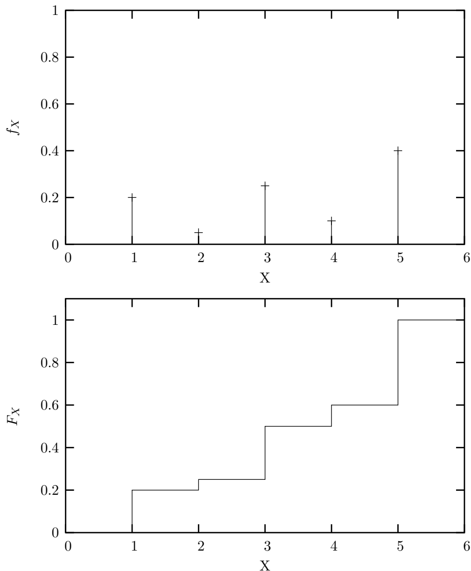
Figura 1: Distribuzione discreta
