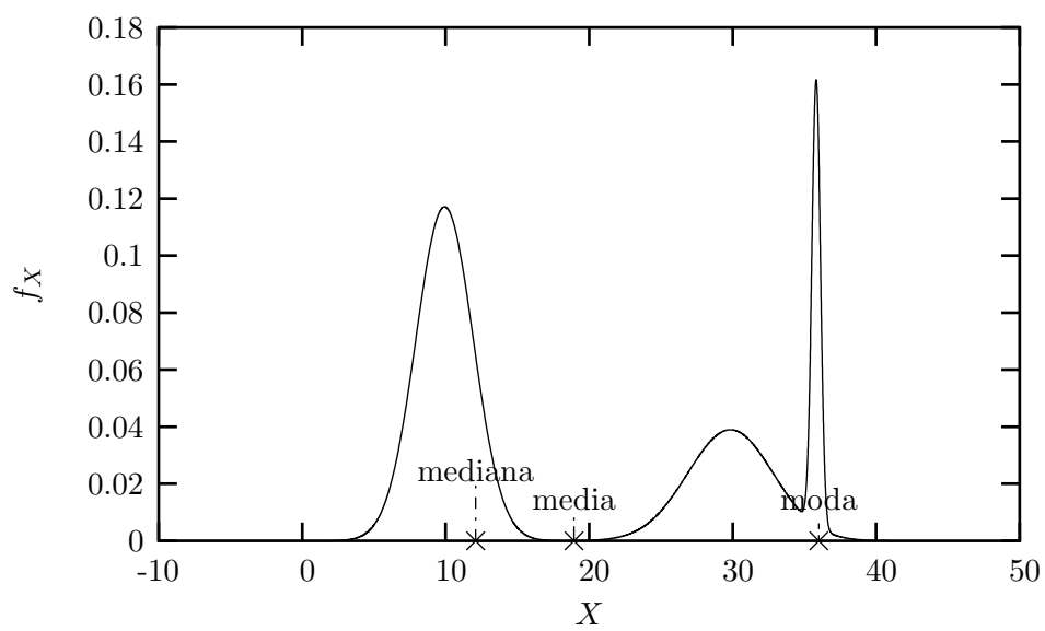
Figura 5: Media, mediana, moda
