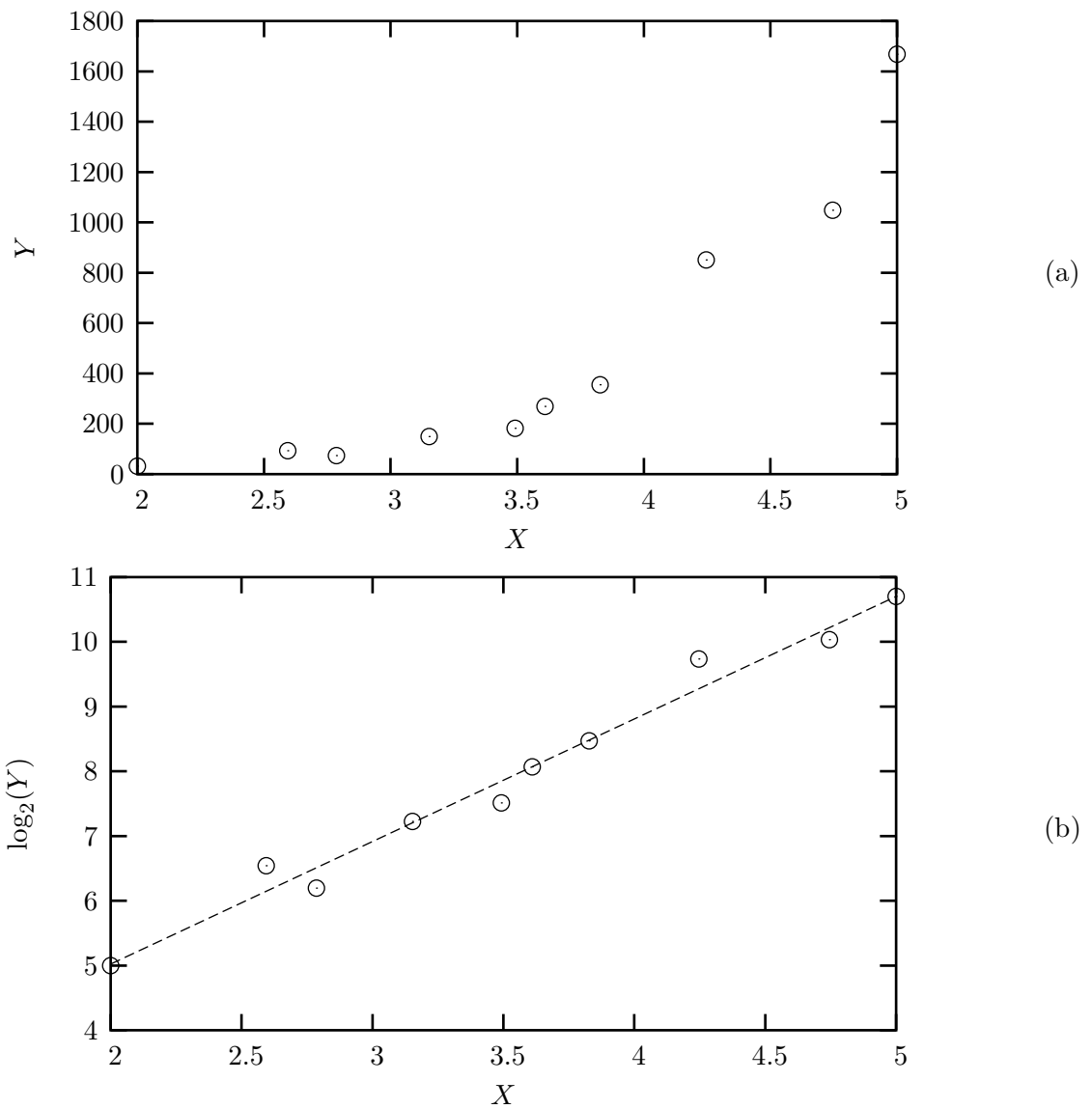
Figura 9: Esempio di un problema di regressione non lineare.
