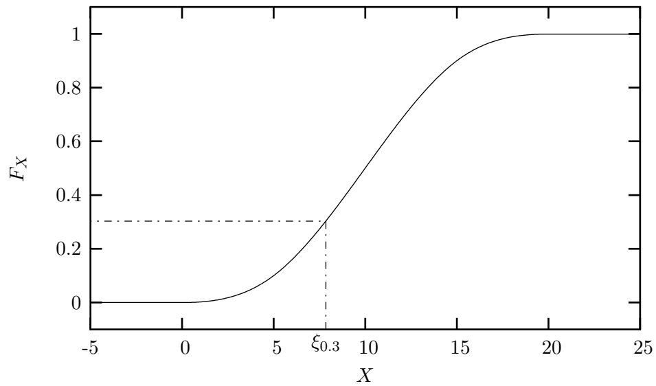
Figura 4: Quantile
